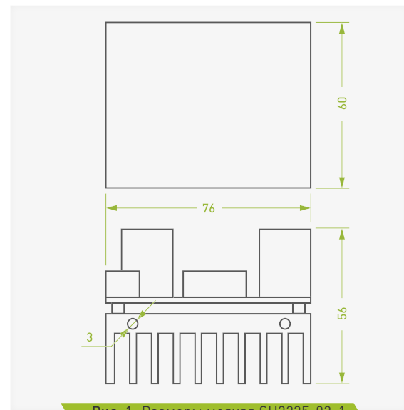
Рис. 1. Размеры модуля SU3235-02-1
