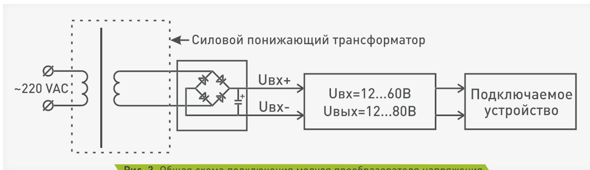
Рис. 3. Общая схема подключения модуля преобразователя напряжения
