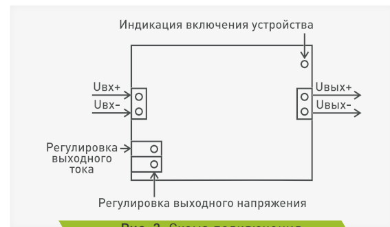
Рис. 2. Схема подключения
