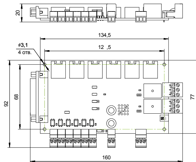
Рис. 1. Размеры устройства коммутации PLC6x-G2
