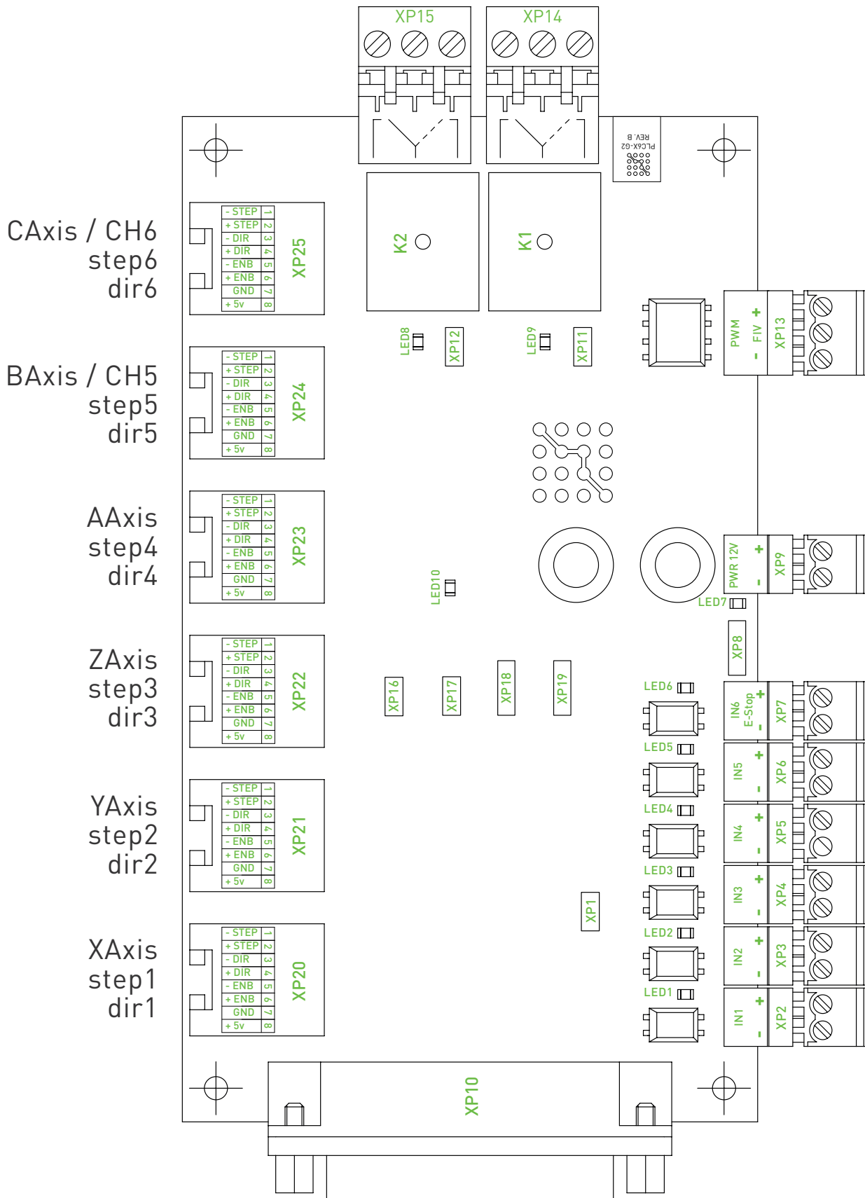
Рис. 2. Назначение разъёмов, переключателей и индикации
