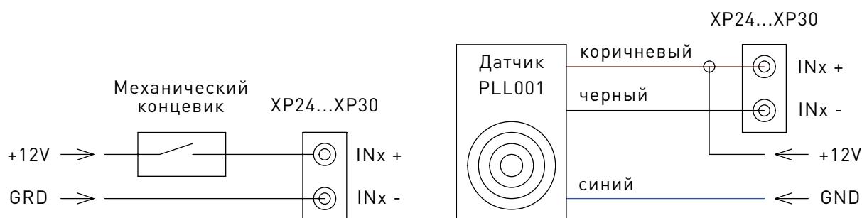
Рис. 6. Подключение концевых датчиков
