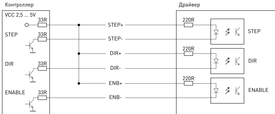
Рис. 5. Устройство выходов контроллера
