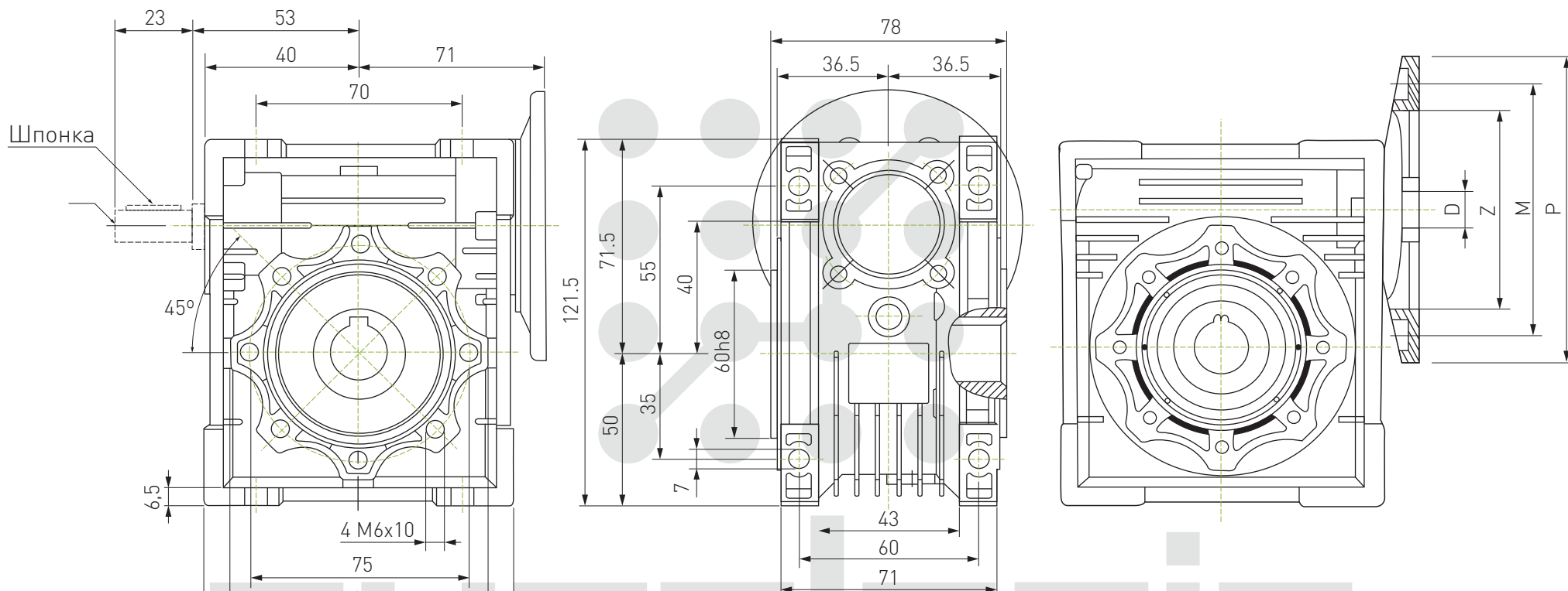
Параметры зубчатого зацепления
