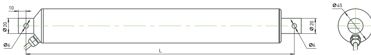
Рисунок 1 – Габаритные и присоединительные размеры (мм) актуаторов TGE.
