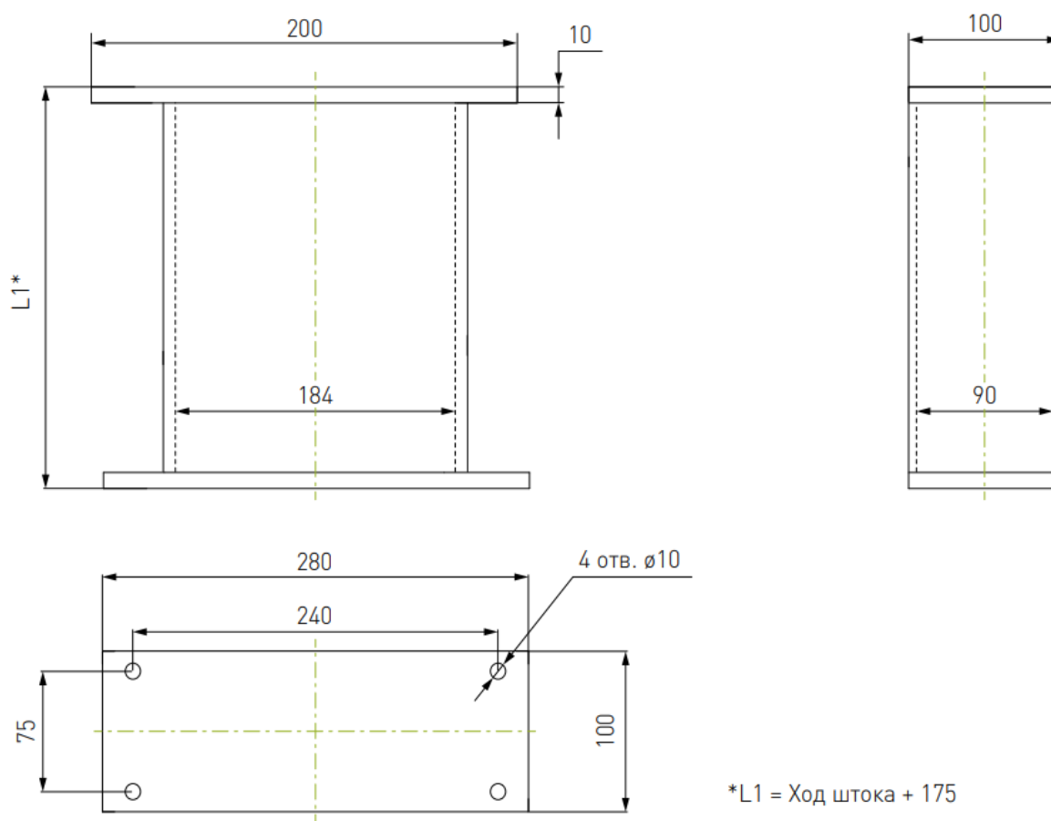
Рисунок 1 – Габаритные и присоединительные размеры (мм) актуаторов TGH-01.
