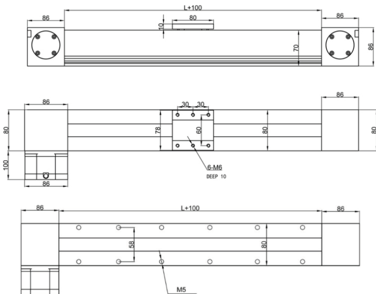
Рисунок 1 – Габаритный чертеж.
