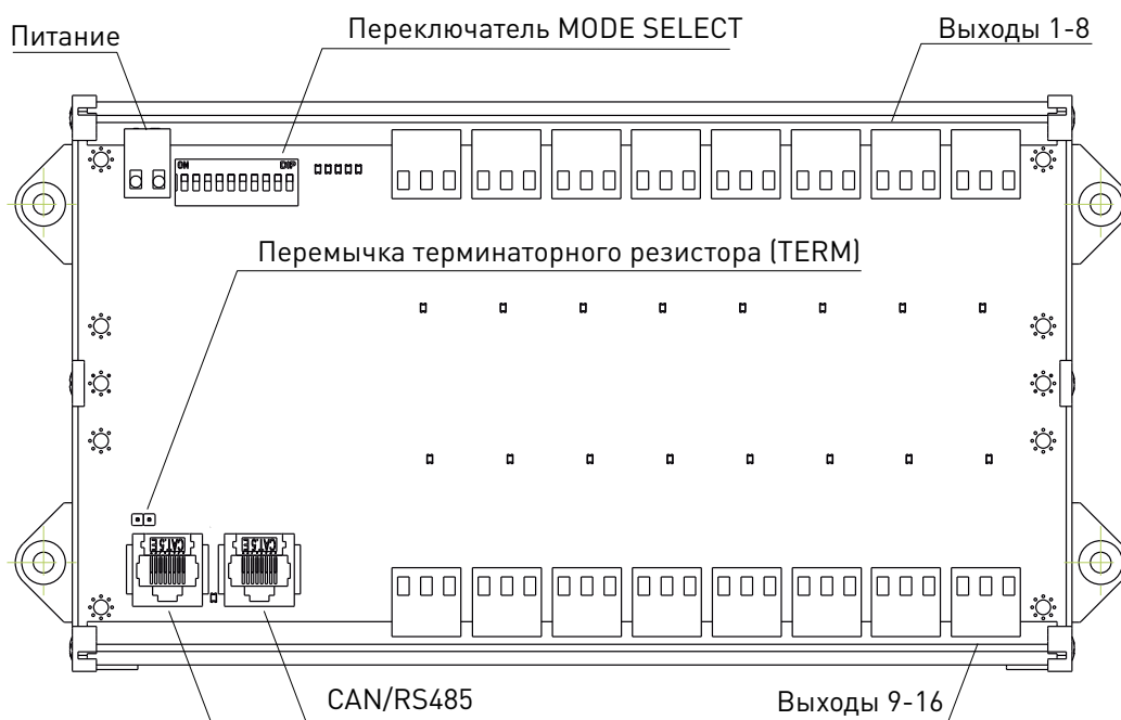
Рисунок 11 — Расположение разъёмов и перемычек PLP-16R-CAN/RS485, PLP-16T-CAN/RS485.
