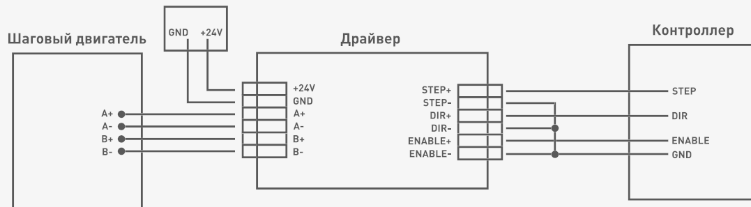
Рис. 6. Общая схема подключения драйвера через контроллер. Управляющие сигналы подключены с общим минусом
