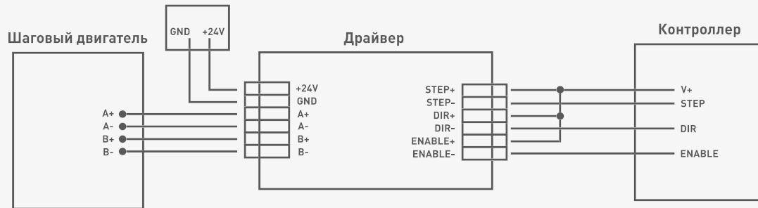
Рис. 5. Общая схема подключения драйвера через контроллер. Управляющие сигналы подключены с общим плюсом
