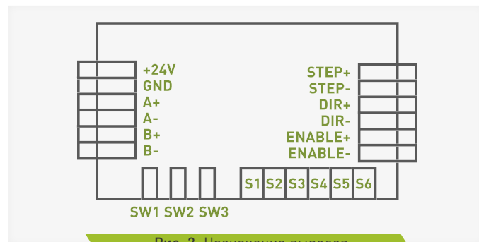
Рис. 2. Назначение выводов
