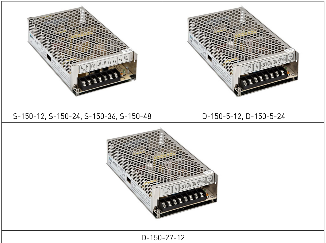
Рис. 1. Внешний вид источников питания
