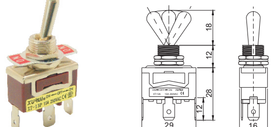
• 单极双投中间停型 SPDT ON-OFF-ON XT-13A
