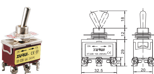
• 双极双投型 DPDT ON-ON XT-22B
