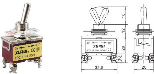
• 双极单投型 DPST ON-OFF XT-21B
