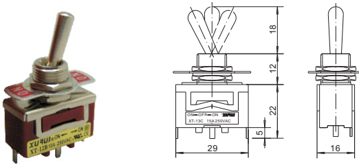
• 单极双投中间停型 SPDT ON-OFF-ON XT-13C
