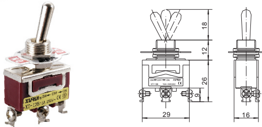
• 单极双投中间停型 SPDT ON-OFF-ON XT-13B
