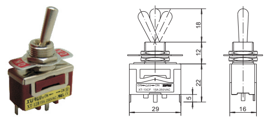
• 单极双向自动复位型 SPDT Auto Reset (ON) -OFF-(ON) XT-13CF
