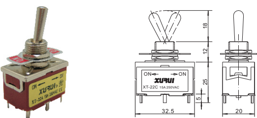
• 双极双投型 DPDT ON-ON XT-22C
