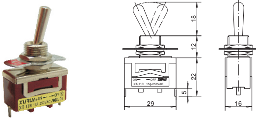
• 单极单投型 SPST ON-OFF XT-11C
