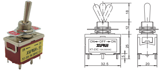
• 双极双投中间停型 DPDT ON-OFF-ON XT-23C
