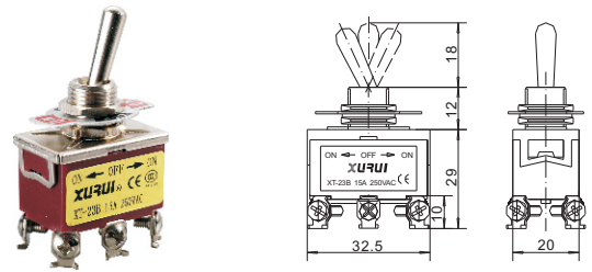
• 双极双投中间停型 DPDT ON-OFF-ON XT-23B
