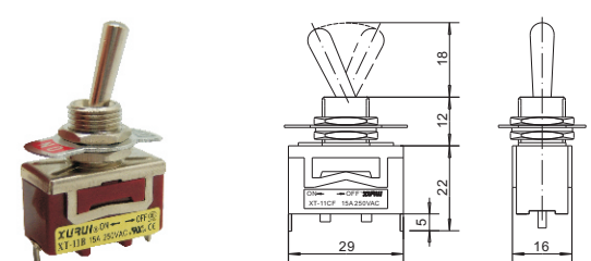
• 单极单向自动复位型 SPST Auto Reset (ON) -OFF XT-11CF
