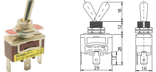
• 单极双投型 SPDT ON-ON XT-12A
