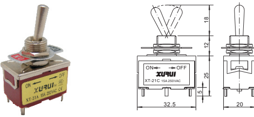
• 双极单投型 DPST ON-OFF XT-21C
