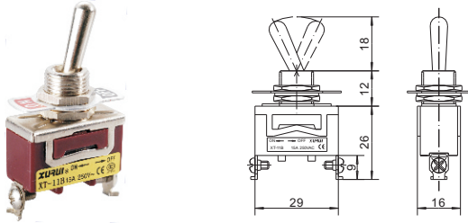
• 单极单投型 SPST ON-OFF XT-11B
