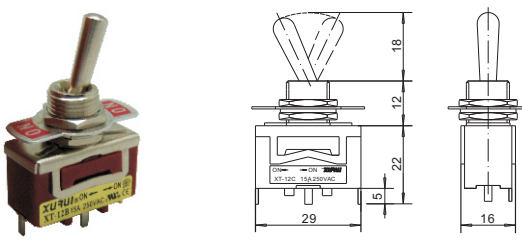
• 单极双投型 SPDT ON-ON XT-12C
