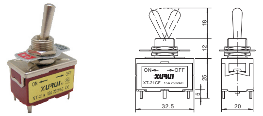
• 双极单向自动复位型 DPST Auto Reset (ON) -OFF XT-21CF
