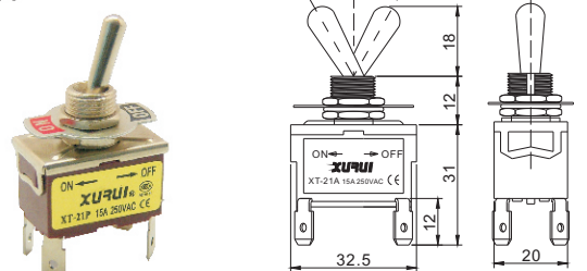
• 双极单投型 DPST ON-OFF XT-21A
