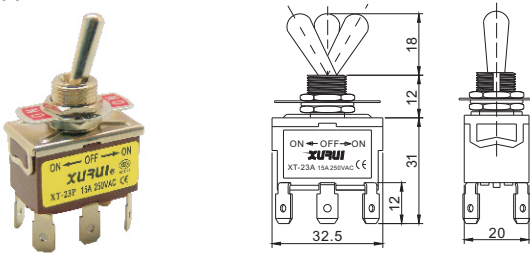
• 双极双投中间停型 DPDT ON-OFF-ON XT-23A
