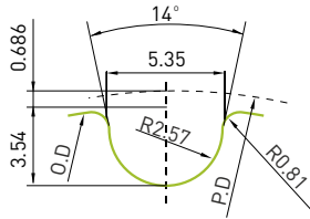
Чертеж профиля зуба шкива 8М
