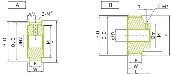
Типы зубчатых шкивов
